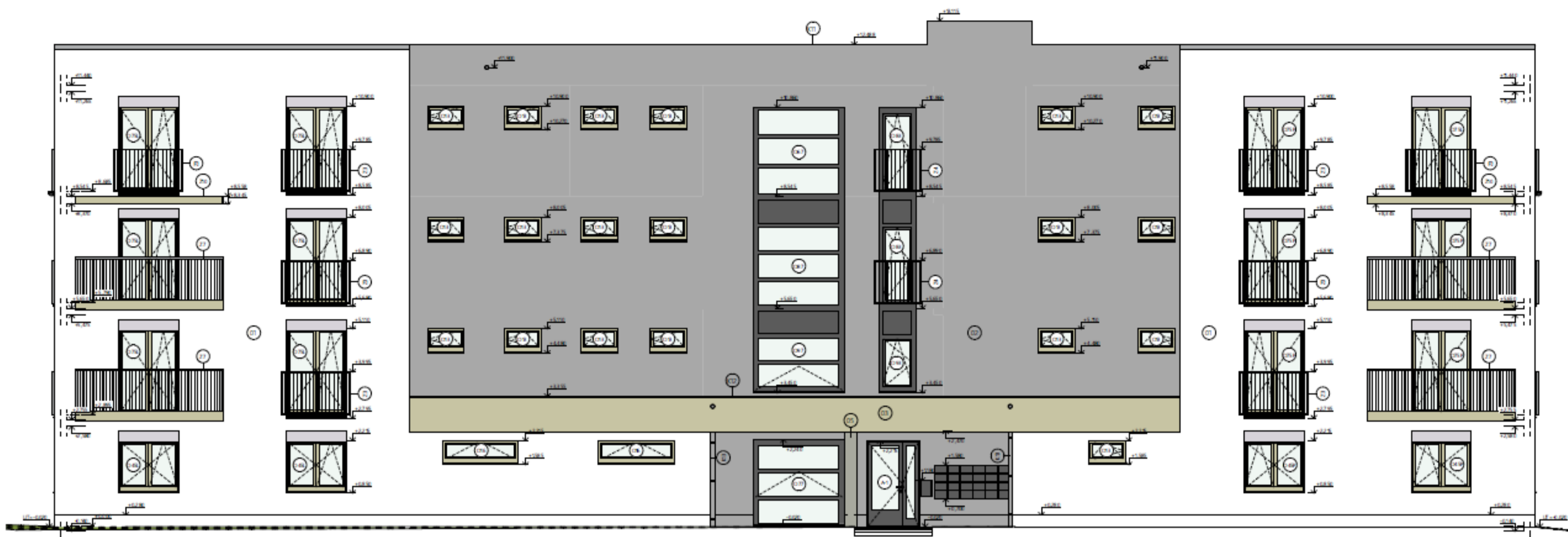
pohled severní
